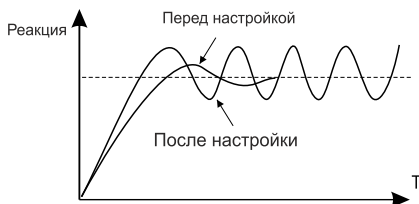
Рис. 6.22 - Контроль вибрации повышенной частоты
