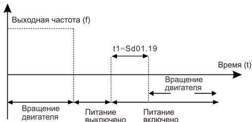
Рис. 6.4 - Автозапуск после отключения питания
