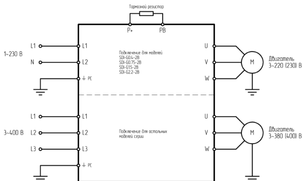
Рис. 3.2 - Схема силовых подключений
