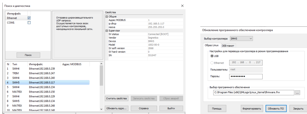
Рис. 56 – Обновление ПО
